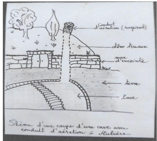
Schéma d'une coupe d'une cave avec conduit d'aération à Aubière
